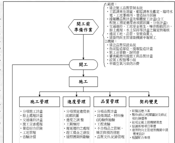
公共工程施工驗收作業程序流程圖(1)
