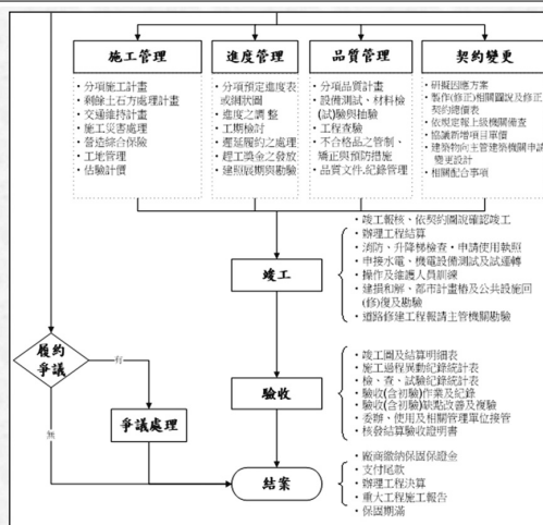
公共工程施工驗收作業程序流程圖(2)
